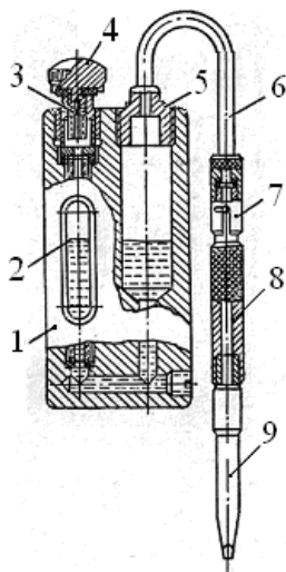
Рис. 1. Принципиальная схема прибора КИ – 4870 ГОСНИТИ
